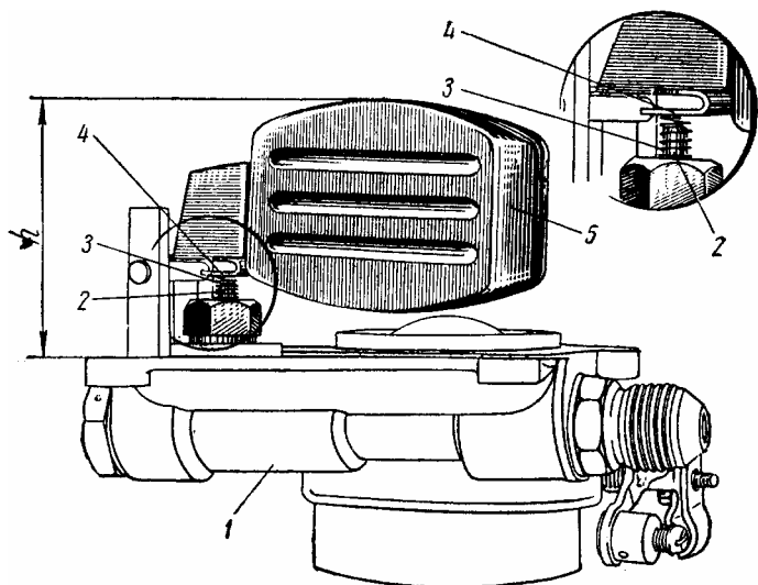
Рис. 23. Проверка правильности положения поплавка
