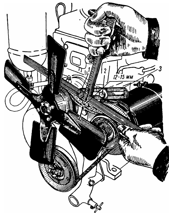
Рис. 20. Проверка натяжения приводного ремня вентилятора
