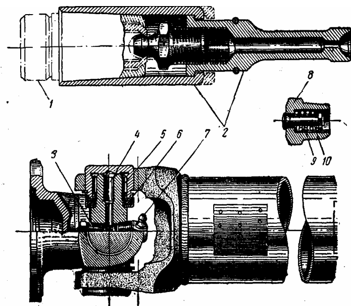
Рис. 27. Расположение пресс-масленки и предохранительного клапана на крестовине карданного шарнира:
