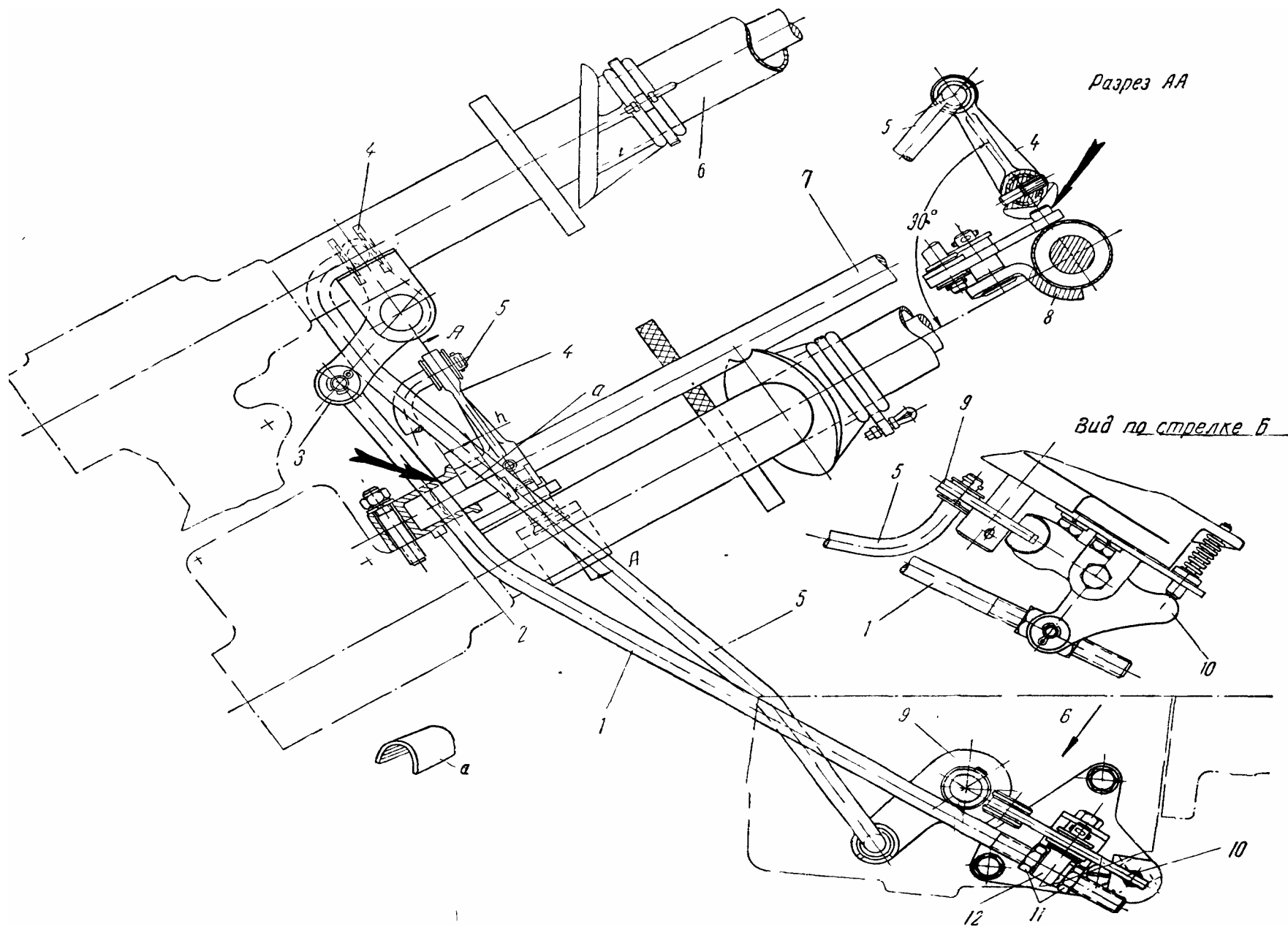
Рис. 26. Механизм привода управления коробкой передач:
