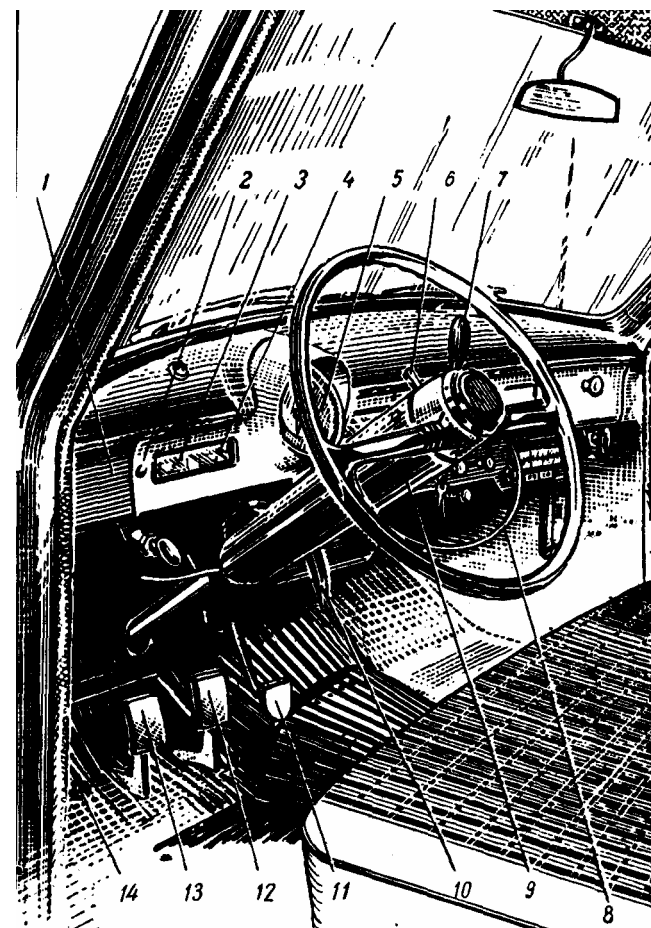
Рис. 4. Органы управления и контрольно-измерительные приборы: 1— панель приборов; 2 — щиток приборов; 3 — амперметр; 4 — указатель уровня бензина в баке; 5 — спидометр; 6 — рычажок переключателя указателей поворотов; 7 — рычаг переключения передач; 8 — включатель звукового сигнала; 9 — кожух рулевой колонки; 10 — вытяжная рукоятка ручного тормоза; 11 — педаль управления дроссельной заслонкой карбюратора; 12— педаль тормоза; 13— педаль сцепления; 14 — кнопка ногожного переключателя света фар
