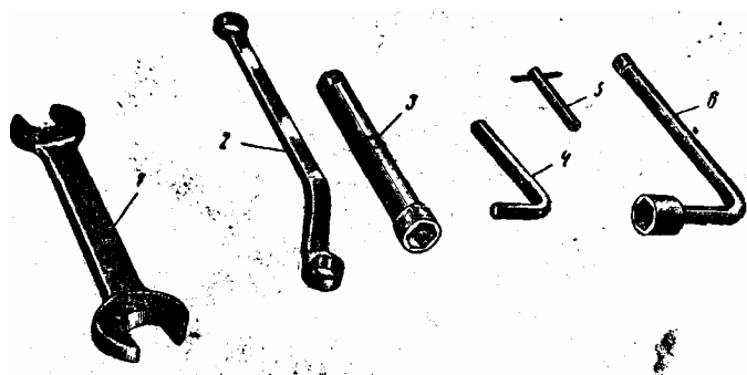
Рис. 43. Специальные ключи, входящие в комплект шоферского инструмента, прилагаемого к автомобилю:
