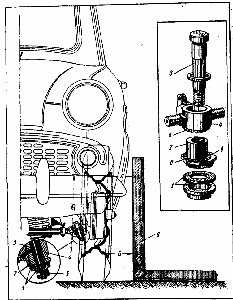
Рис. 35. Проверка угла развала переднего колеса
