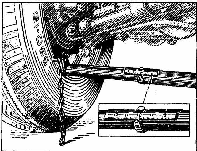
Рис. 33. Проверка схождения передних колес
