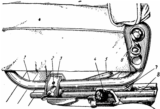
Рис. 8. Салазки перемещения переднего сиденья
