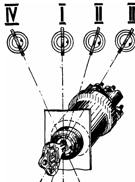
Рис. 7. Положения ключа в замке зажигания:
