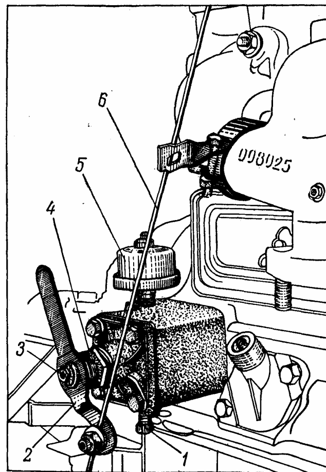
Рис. 14. Установка фильтра грубой очистки масла на двигателе
