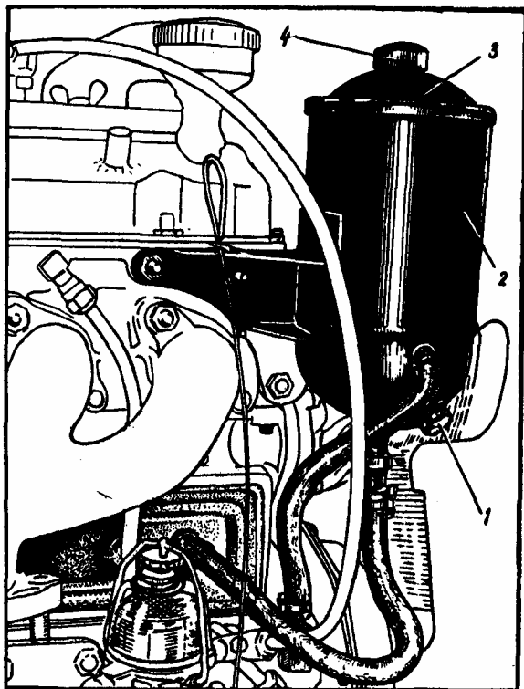
Рис. 15. Установка фильтра тонкой очистки масла на двигателе
