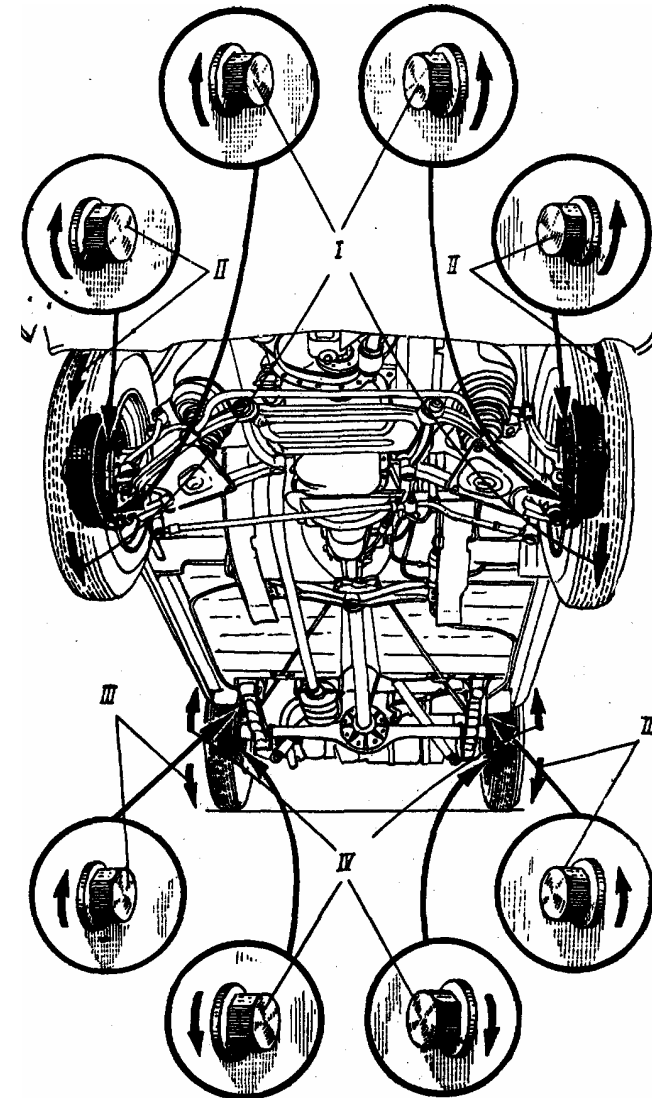
Рис. 38. Направление вращения регулировочных эксцентриков и колес автомобиля при регулировке тормозов:
