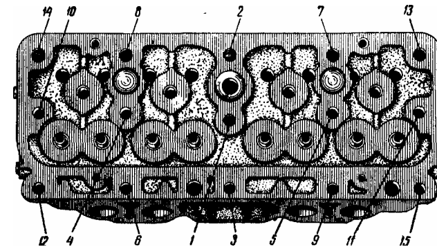
Рис. 19. Последовательность затяжки болтов крепления головки блока цилиндров к блоку
