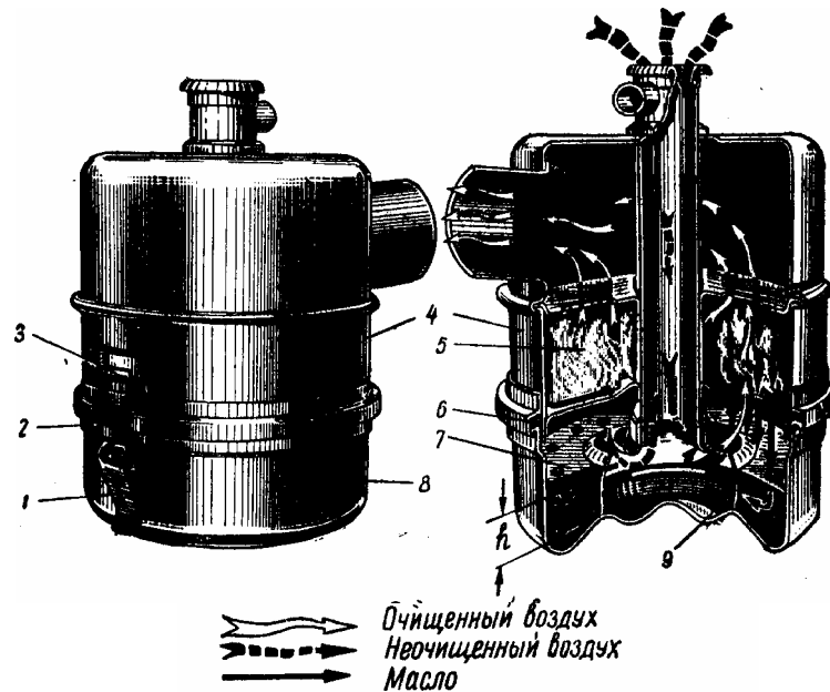
Рис. 16. Воздухоочиститель
