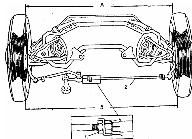
Рис. 34. Размеры, определяющие схождение передних колес
