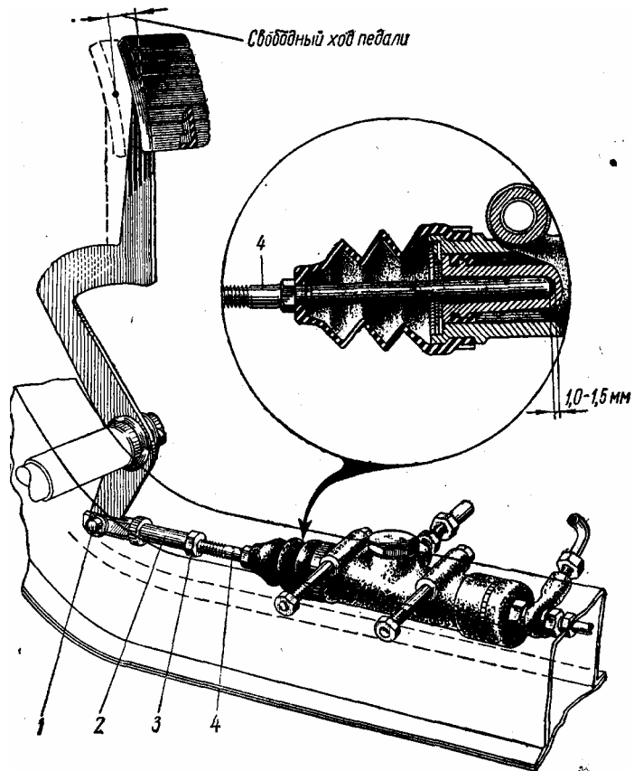
Рис. 37. Регулировочный узел гидравлического привода ножного тормоза: 1 — шарнирный палец; 2 — вилка толкателя; 3 — контргайка; 4 — толкатель
