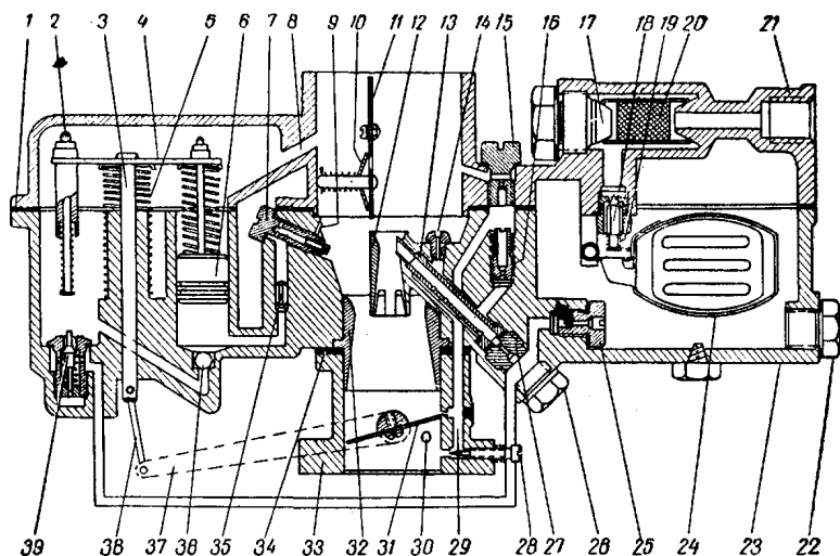
Рис. 21. Схема карбюратора типа К-59:
