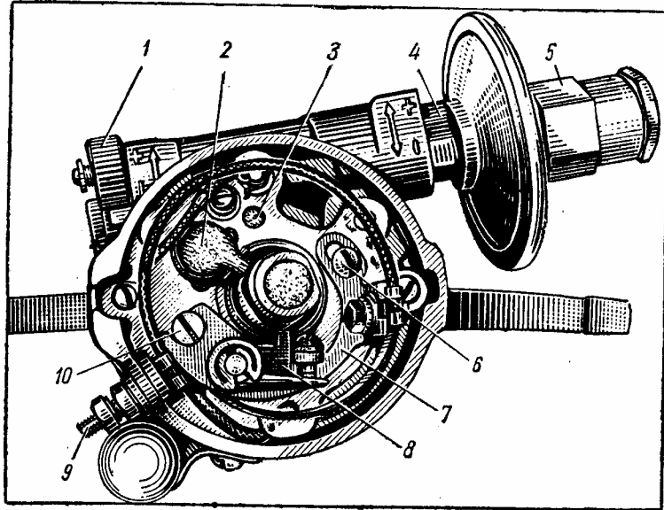
Рис. 24. Распределитель зажигания (со снятыми крышкой и ротором)
