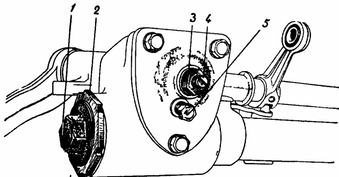
Рис. 36. Регулировочные устройства рулевого механизма
