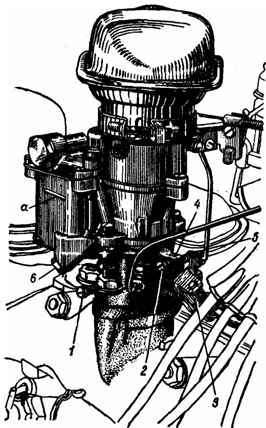
Рис. 22. Винты карбюратора для регулировки состава смеси холостого хода двигателя
