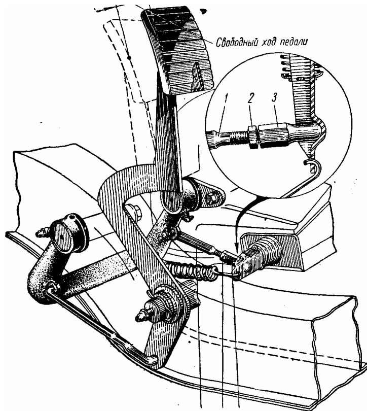
Рис. 25. Регулировочный узел привода выключения сцепления
