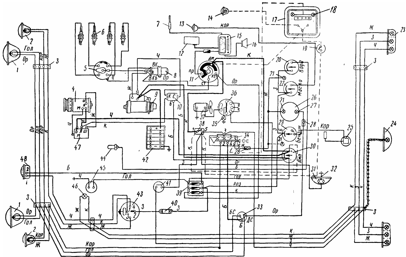
Рис. 41. Схема электрооборудования:
