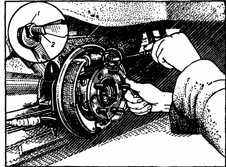
Рис. 39. Регулировка положения разжимного рычага на задней колодке тормоза
