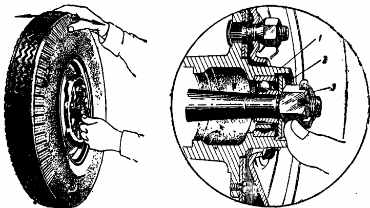
Рис. 28. Проверка подтяжки подшипников ступицы переднего колеса
