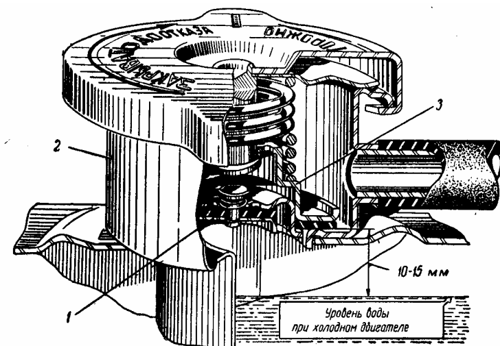
Рис. 13. Наполнительная горловина радиатора с установленной пробкой: 1 — воздушный клапан; 2 — горловина; 3 — паровой клапан
