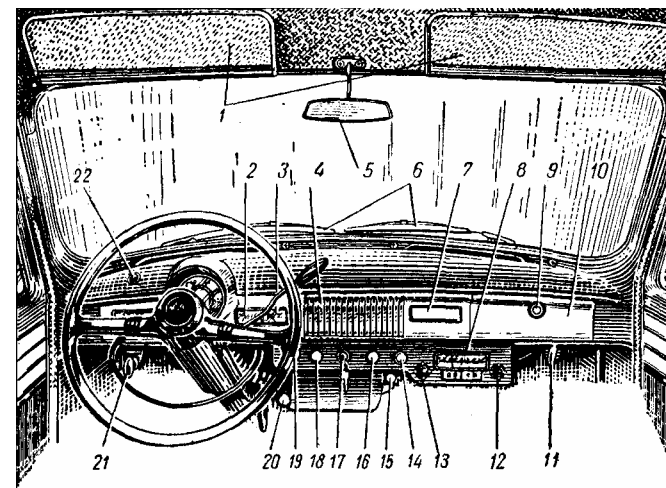
Рис. 6. Панель приборов и оборудование места шофера:
