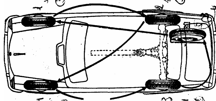
Рис- 29. Схема перестановки колес
