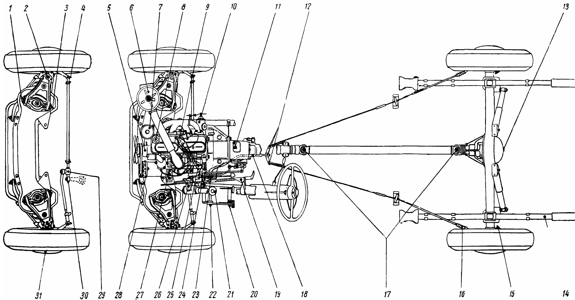
Рис 11. Карта смазки механизмов шасси автомобиля
