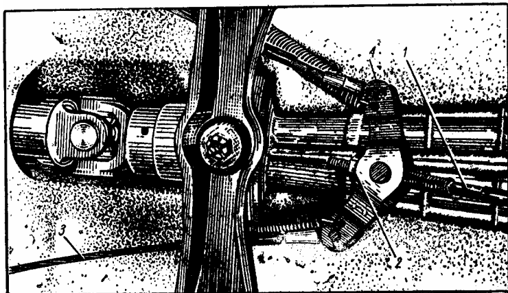
Рис. 40. Регулировочный узел механического привода ручного тормоза
