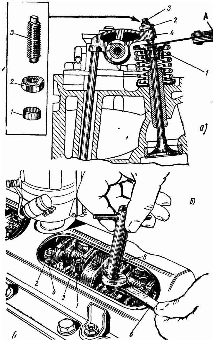
Рис 17. Проверка и регулировка зазора между нажимным болтом коромысла и наконечником стержня клапана: а — проверка; б — регулировка
