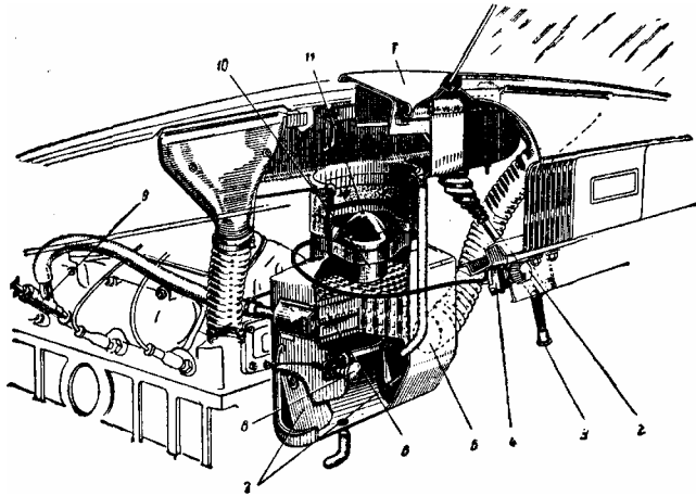
Рис. 10. Отопитель кузова и обогреватель ветрового стекла
