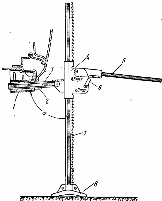
Рис. 30. Установка домкрата для вывешивания колеса автомобиля
