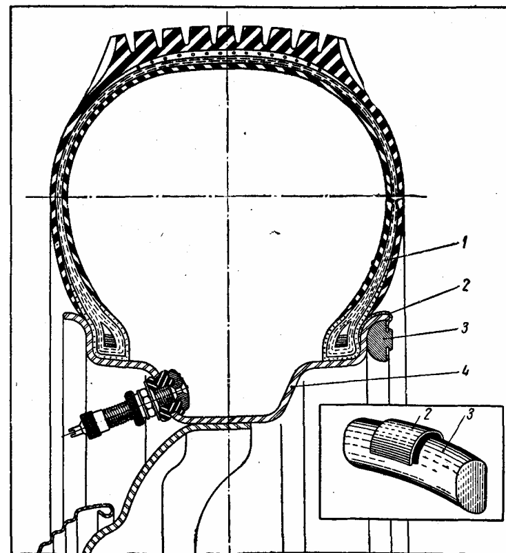
Рис. 31. Крепление балансировочного грузика на ободу колеса
